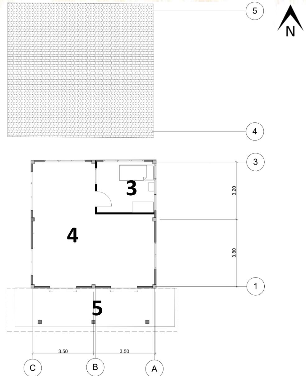
แปลนชั้น 2
