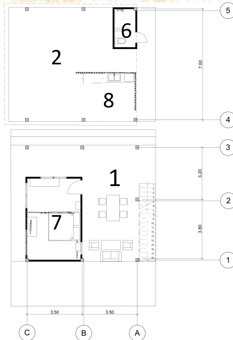
แปลนชั้น 1
